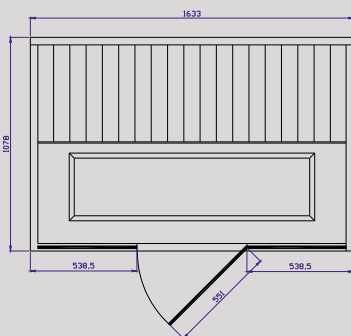
TYLÖSAND T-825 Maße: T 1078 x B 1633 mm
