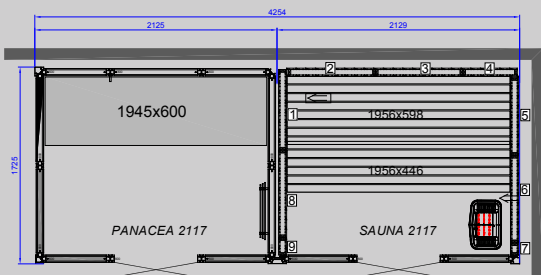
TWIN PANACEA 2117 Maße: T 1725 x B 4254 mm
