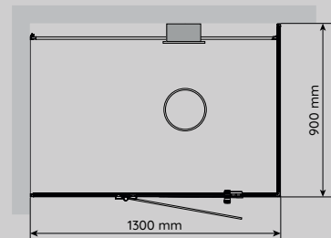
VISTA 130 RECHTS Maße: T 900 x B 1300 mm
