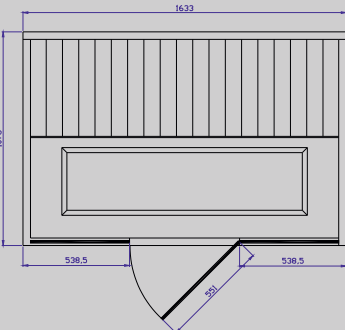
TYLÖSAND T-825 Maße: T 1078 x B 1633
