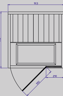
TYLÖSAND T-810 Maße: T 913 x B 913 mm
