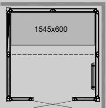
PANACEA 1717 1B Maße: 1725 x 1725 x 2090 mm
