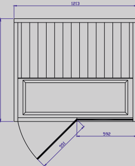
TYLÖSAND T-820 Maße: T 1013 x B 1213 mm
