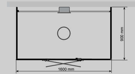
VISTA DCO 160 (LINKS & RECHTS) Maße: T 900 x B 1600 mm
