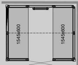
PANACEA 2117 2B Maße: 2125 x 1725 x 2090 mm
