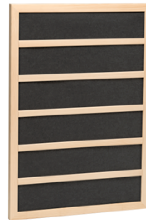
Leistung 300 W B 680 × T 37 × H 980 mm
