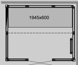
PANACEA 2117 1B Maße: 2125 x 1725 x 2090 mm
