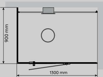
VISTA 130 LINKS Maße: T 900 x B 1300 mm
