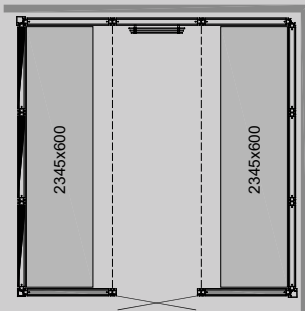
PANACEA 2525 2B Maße: 2525 x 2525 x 2090 mm
