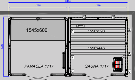
TWIN PANACEA 1717 Maße: T 1725 x B 3454 mm
