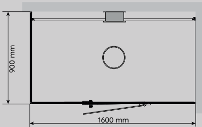
VISTA 160 LINKS Maße: T 900 x B 1600 mm
