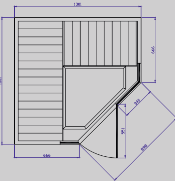
TYLÖSAND T-870 Maße: T 1301 x B 1301 mm
