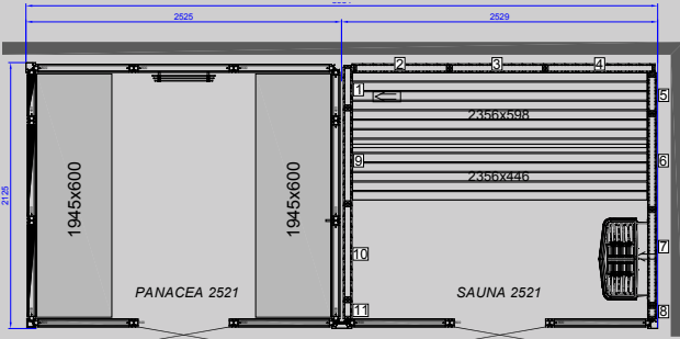
TWIN PANACEA 2521 Maße: T 2125 x B 5054 mm
