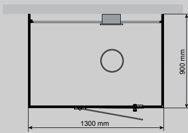
VISTA DCO 130 RECHTS Maße: T 900 x B 1300 mm
